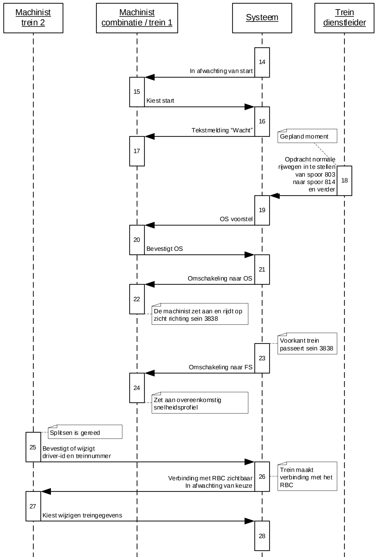
figuur 70 interactie splitsen van een trein, deel 2 vertrek trein 1 en vertreggereedmaken trein 2
