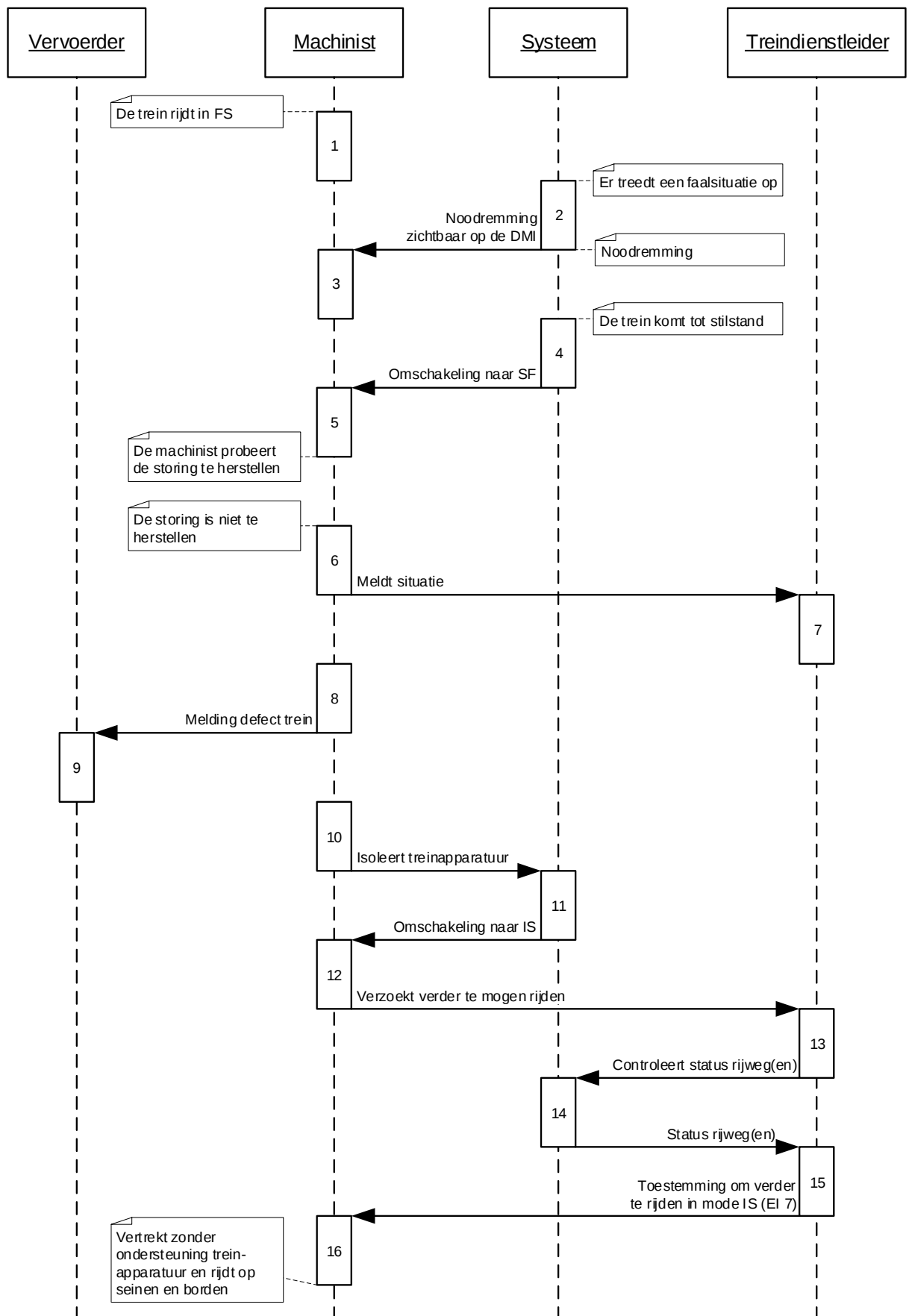
figuur 105 Interactie verder rijden met buiten bedrijf gestelde ETCS apparatuur na treinstoring
