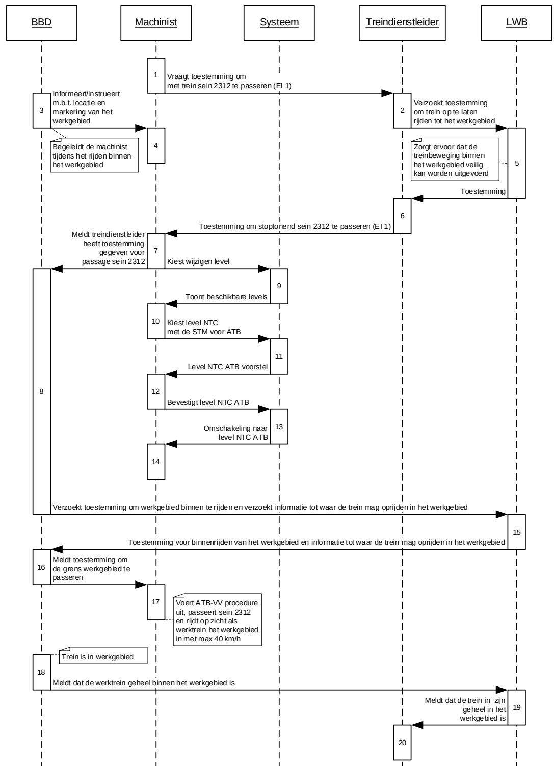
figuur 109 interactie binnenrijden werkgebied met lichtsein op de grens
