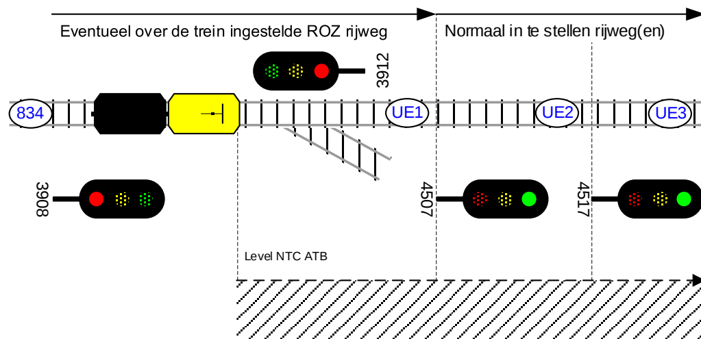
figuur 14 Uitgangssituatie vertrek met wissel tussen trein en sein
