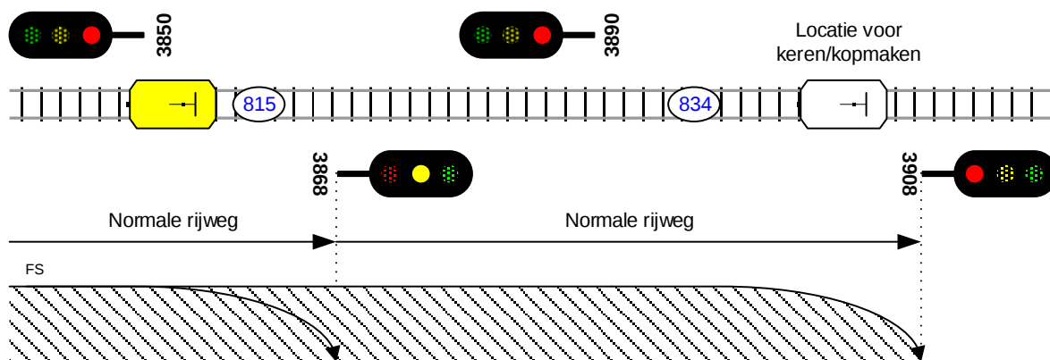
figuur 62 situatie aankomst van de trein voor het keren/kopmaken
