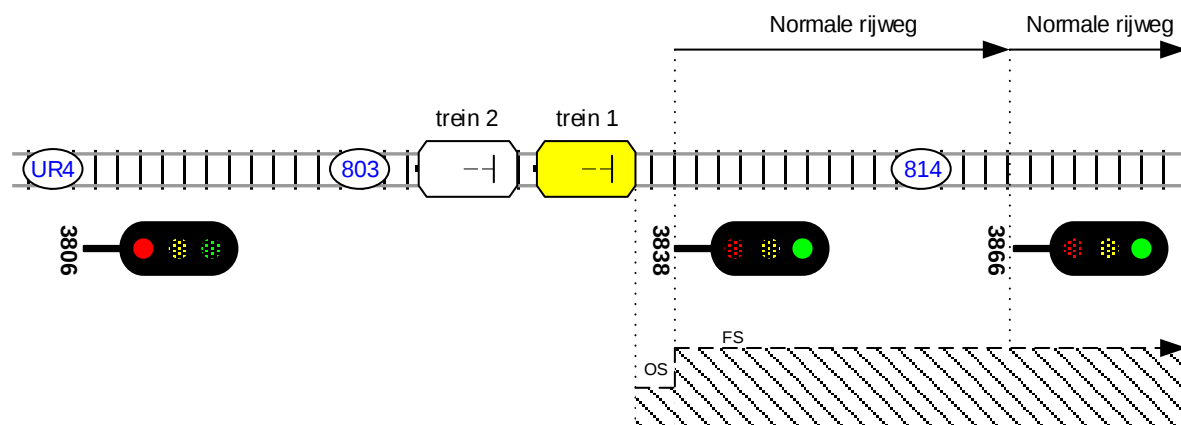
figuur 67 situatie na het splitsen van de treinen, vertrek van trein 1
